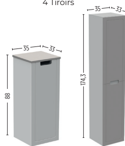
PANADCOL35 D/G
